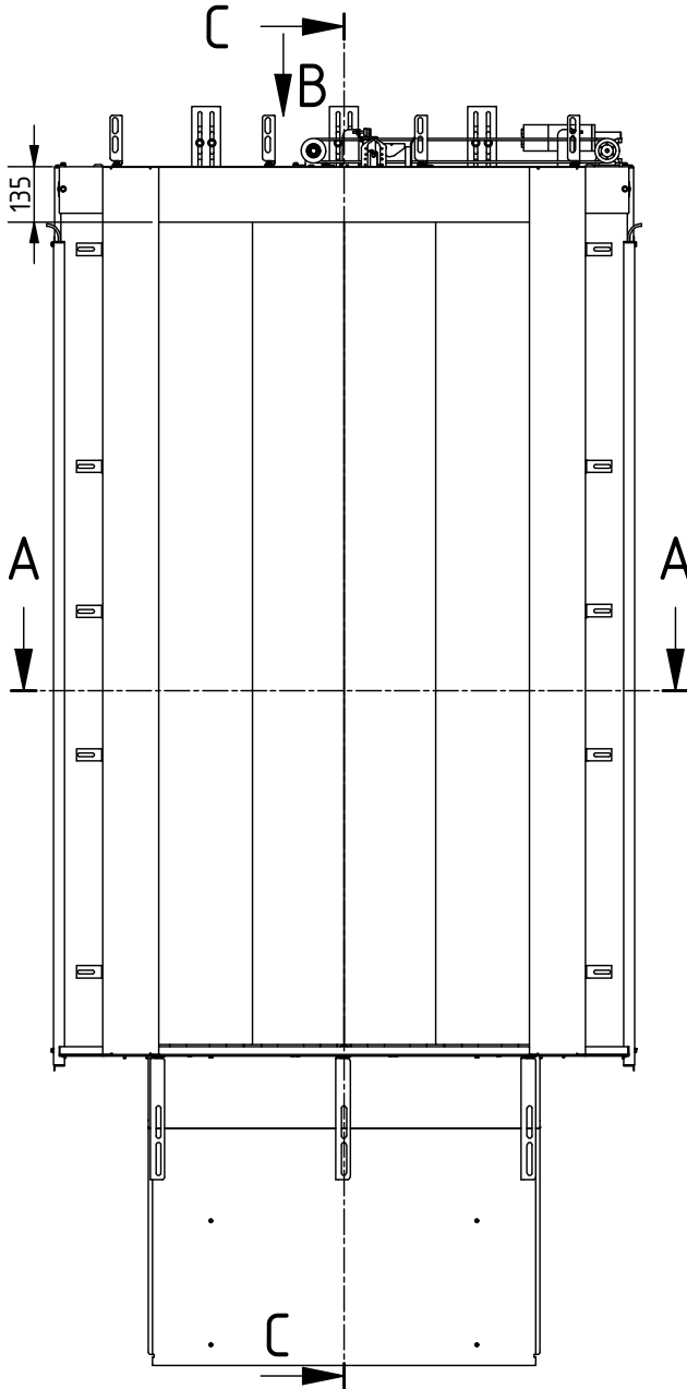
RTZK4 Kabinenschiebetür
