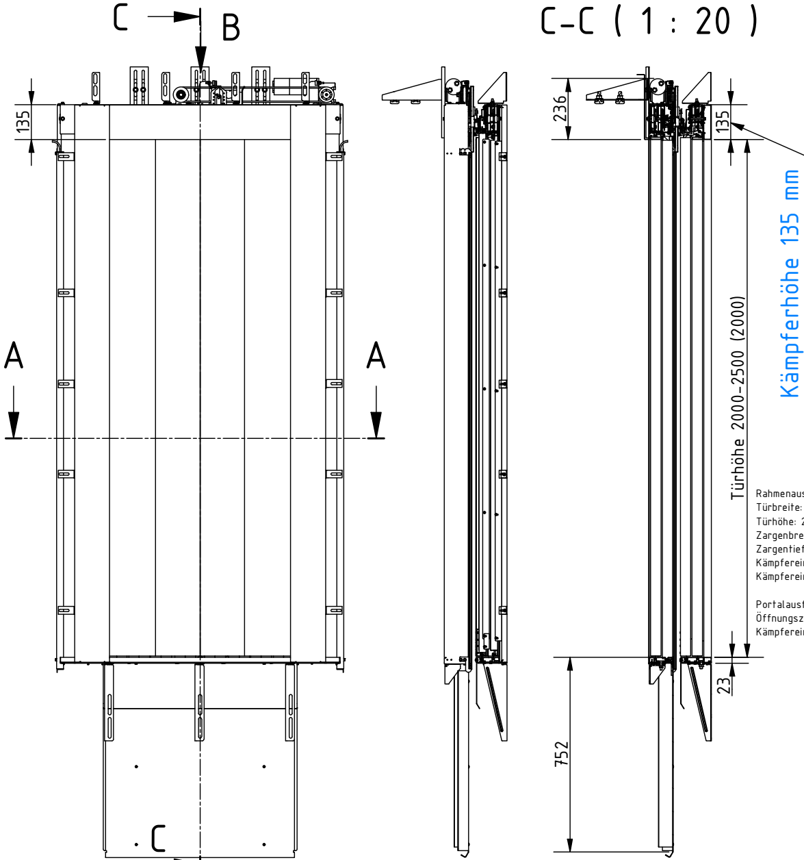
RTZK4 Kabinenschiebetür
