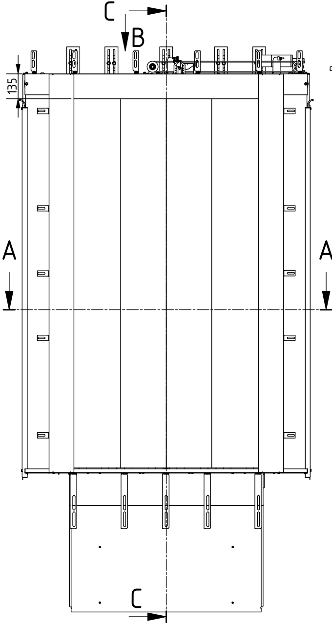
RTZK4 Kabinenschiebetür
