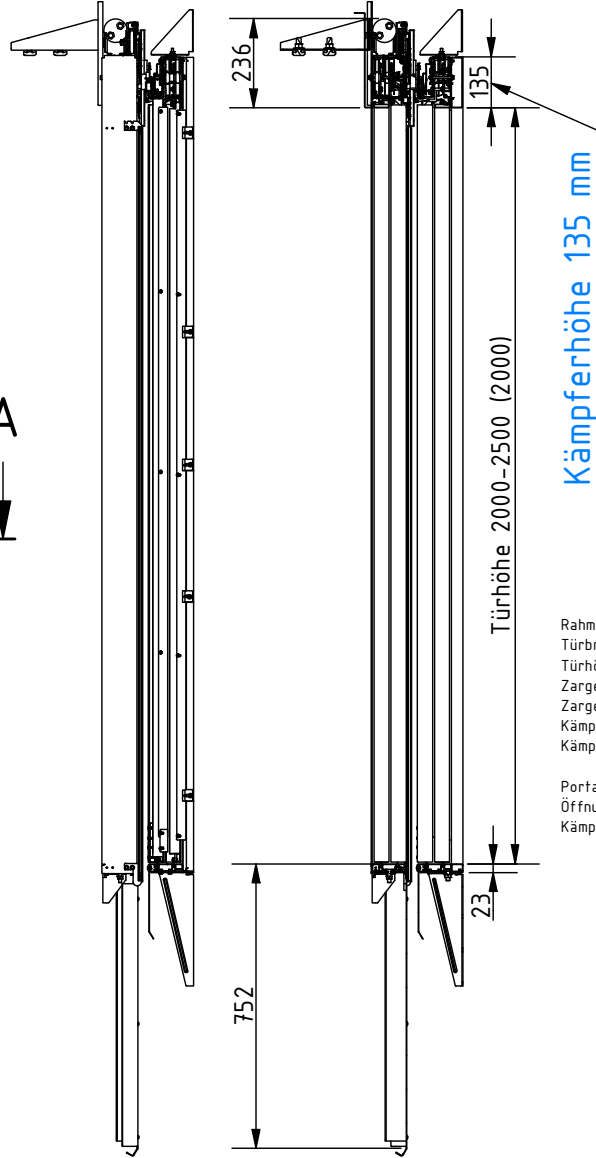
RTZK4 Kabinenschiebetür
